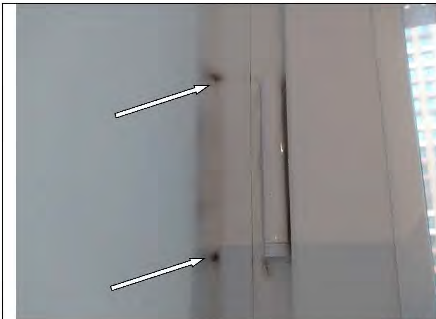
Фото №43. Следы скопления пыли, свидетельствующие об инфильтрации воздуха через петли оконного блока №2 в гостиной.
