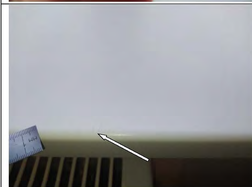
Фото №36. На лицевой поверхности подоконной доски оконного блока №1 в гостиной имеются дефекты (царапины).
