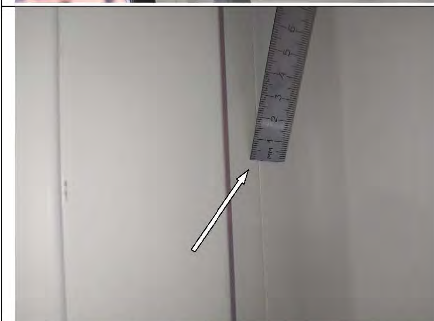
Фото №32. Профиль ПВХ оконного блока №6 в кухне имеет дефекты (царапина).
