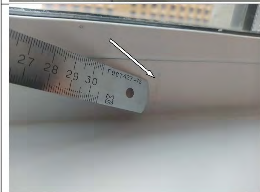
Фото №27. Профиль ПВХ оконного блока №2 в гостиной имеет дефекты (царапины).
