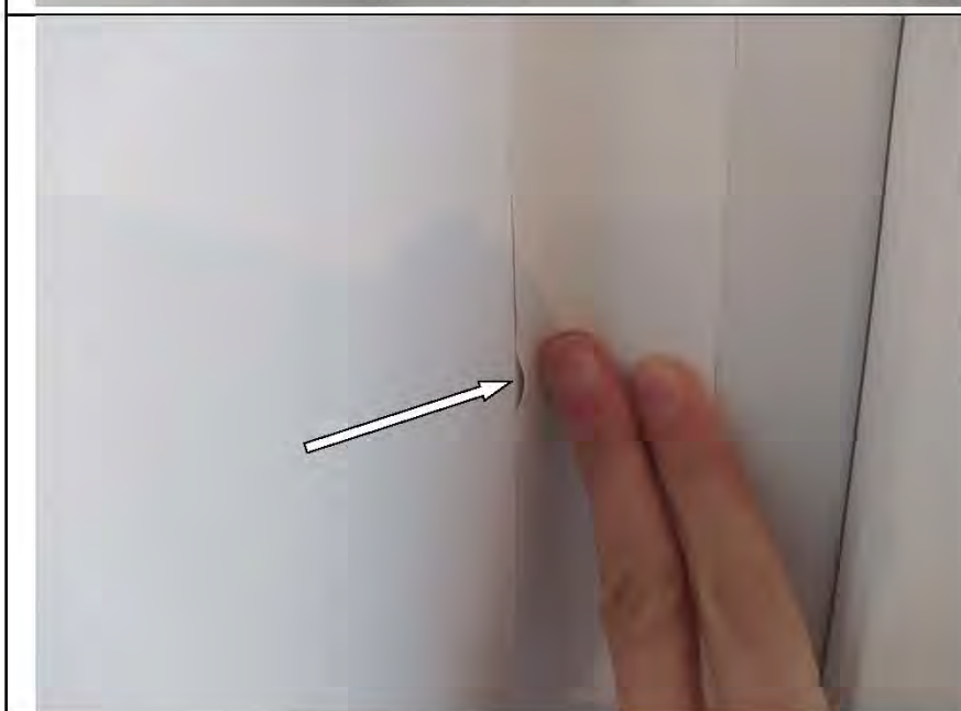
Фото №45. Некачественный монтаж гибкого ПВХ уголка в местах стыков оконного блока №1 с откосами в гостиной (частичное отсутствие герметизирующего состава).
