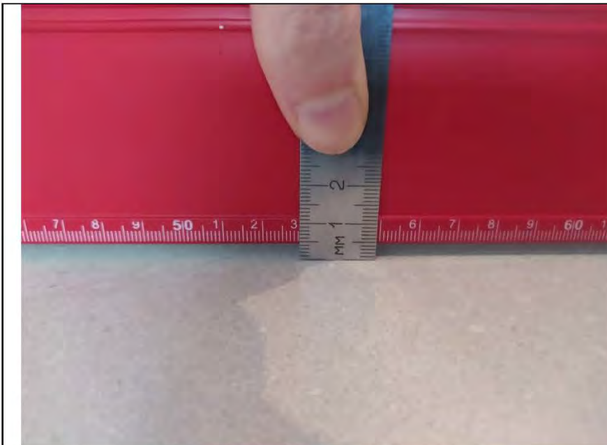
Фото №16. Измерения уровня напольного покрытия в кухне.
