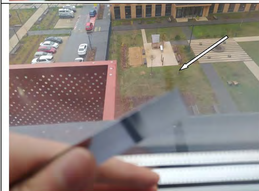
Фото №35. На стеклопакете оконного блока №4 ПВХ в спальне имеется дефект (окалина).
